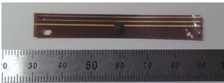
2.45G の RFID タグの中身
